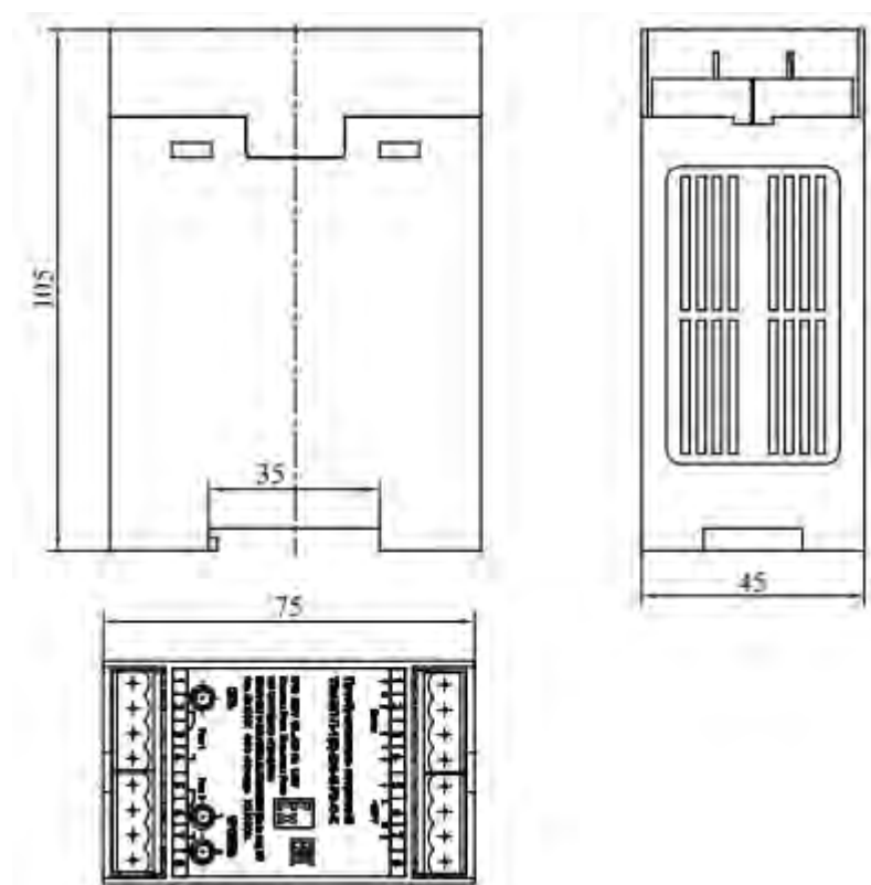
Рисунок Д.1.2 – Габаритные и установочные размеры планки для установки вторичного преобразователя конструктивного исполнения корпуса – настенный алюминиевый.
