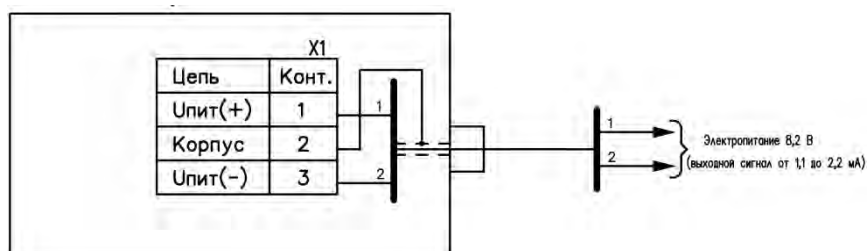
Рисунок Г.2 – Схема электрическая подключения сигнализаторов с выходными сигналами исполнения Natup (к системе верхнего уровня или преобразователю вторичному).
